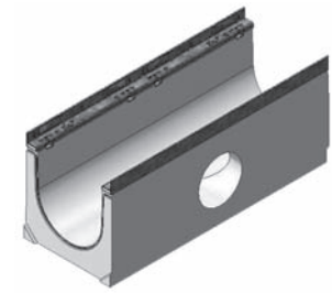
vrtání otvoru DN 200
