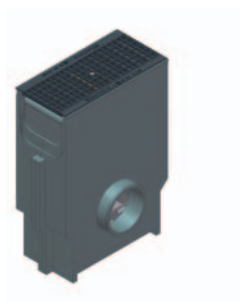
odtoková vpust s pozinkovaným košem, s GUGI litinovým pororoštem oka 20/30, černý, třída C 250
