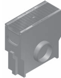
odtoková vpust s pozinkovaným košem, s pororoštem oka 30/10, pozinkovaný, třída B 125
